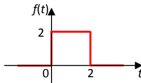
Fig 1. Représentation temporelle de f(t)
