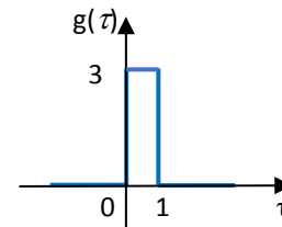
Fig 4. Représentation temporelle de g(\tau)
