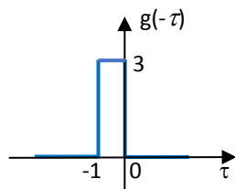
Fig 5. Retournement de g(\tau)
