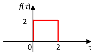
Fig 3. Représentation temporelle de f(\tau)
