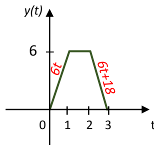
Fig 12. Produit de convolution f * g
