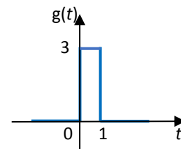
Fig 2. Représentation temporelle de g(t)
