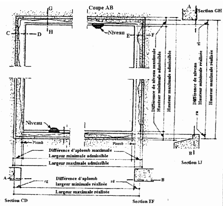
Figure A2.2 Coupe et section verticale et section horizontale Dimension réalisées par rapport aux dimensions admissibles d'une baie
