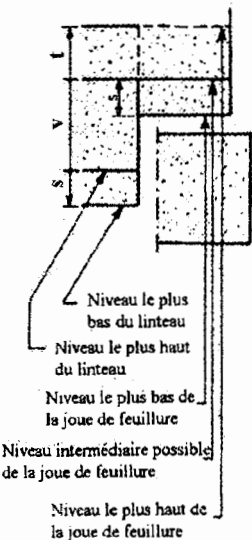
Fig. A2.3b Section d'une feuillure en linteau
