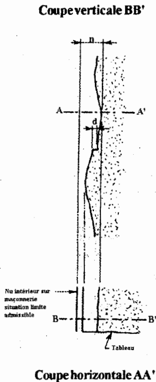
Figure A2.5a : Coupes en tableau sans feuillure
