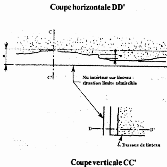
Figure A2.5b : Coupes en linteau sans feuillure
