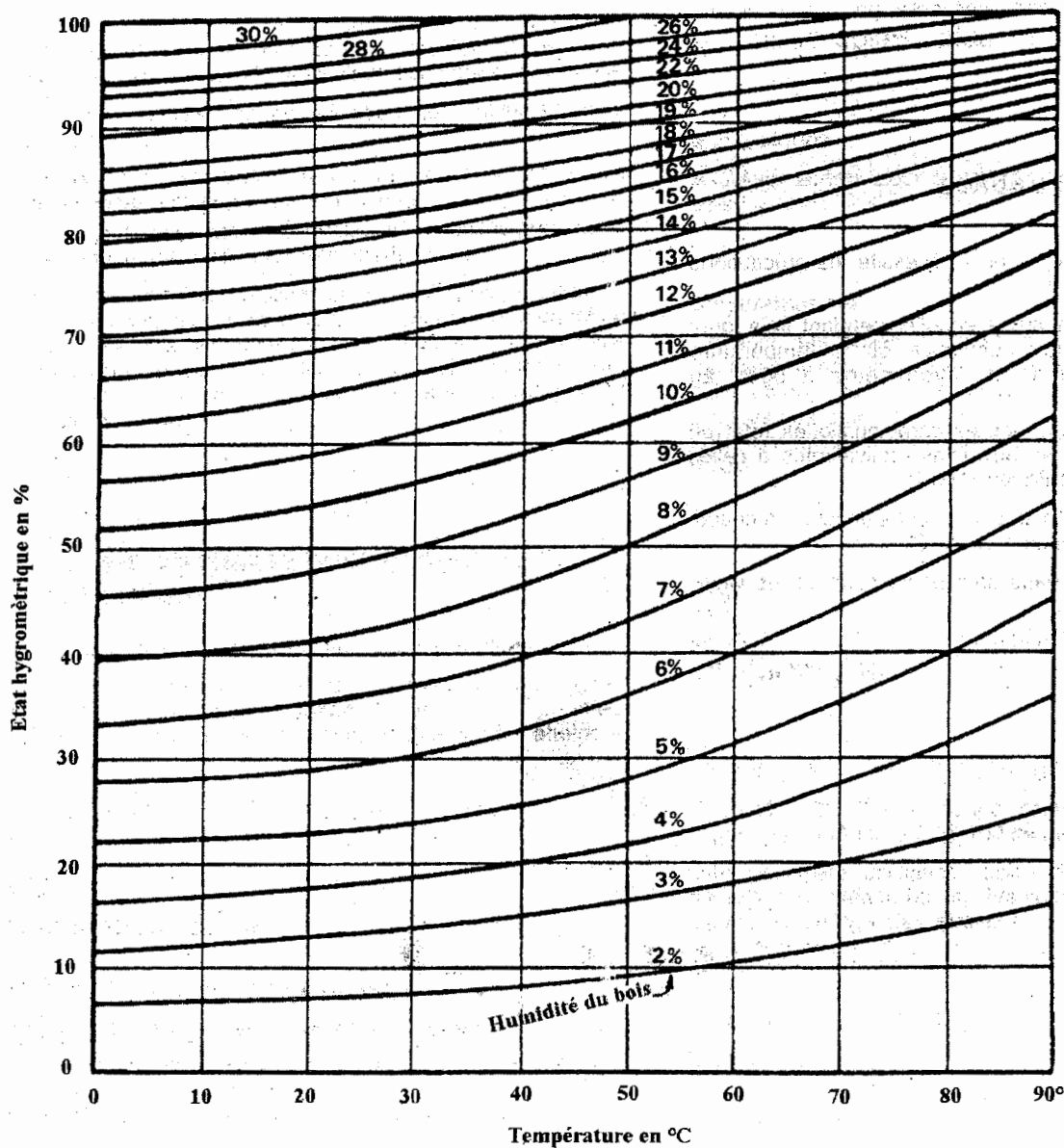
Figure 1 : Courbes d'équilibre hygroscopique du bois
