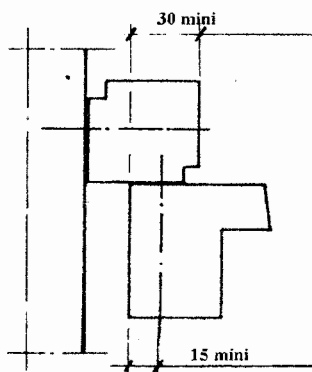
Figure 3 : Profils de jonction
