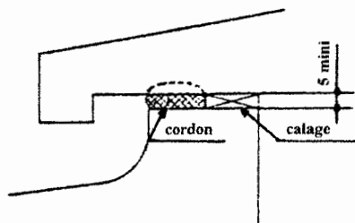
Figure 5 : Calfeutrement avec cordon préformé
