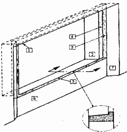
Figure A2.1c Baie avec ébrasement pour pose de la menuiserie en feuillure
