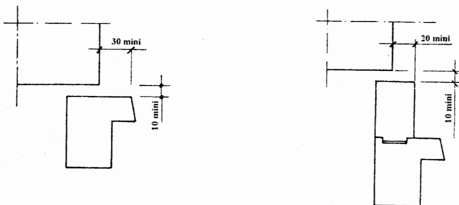
Figures 1 et 2 : Pose avec fourrure d'épaisseur
