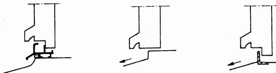
Figure 1 : Etanchéité des seuils
