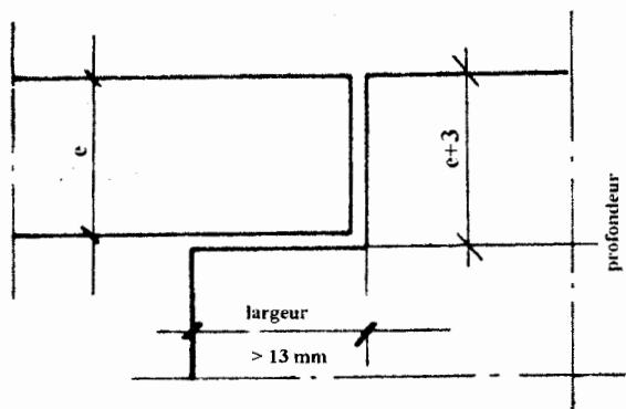
Figure 2 - Portes affleurantes avec huisserie bois
