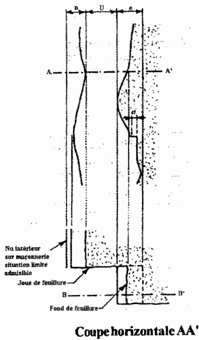
Figure A2.4a : Coupes en tableau avec feuillure
