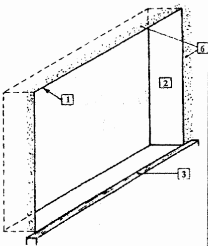
Figure A2.1b Baie pour la pose de la menuiserie en applique intérieure
