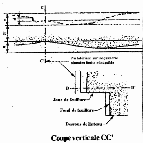
Figure A2.4b : Coupes en linteau avec feuillure
