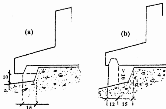
Figure 4 : Etanchéité des pièces d'appui
