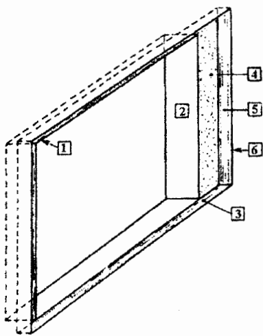
Figure A2.1a Baie pour la pose de menuiserie en feuillure au nu intérieur
