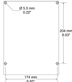
Plans de perçage pour MICROMASTER 420
