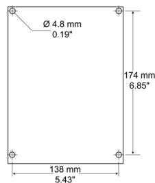
Plans de perçage pour MICROMASTER 420
