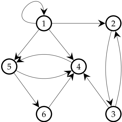
Figure 1.19 : le graphe pour calculer les composantes connexes
