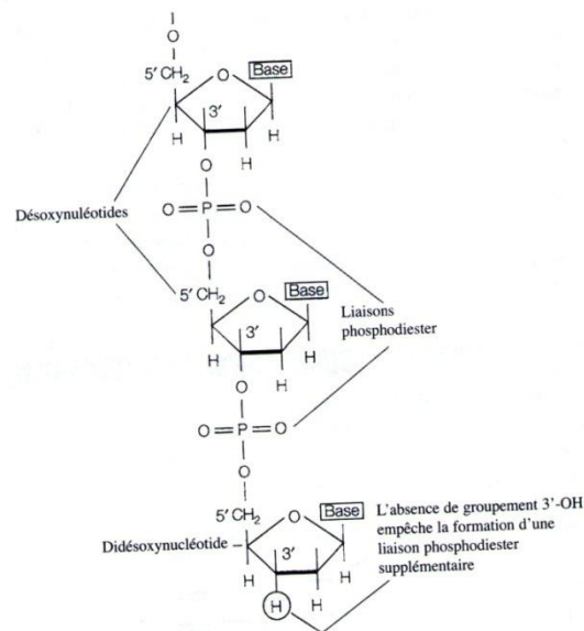
Fig. 1. Terminaison de la synthèse d'ADN par des didésoxynucléotides.
