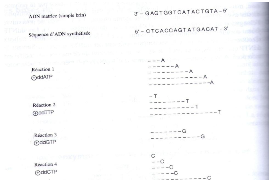
Fig. 2. Séquençage par la méthode enzymatique de terminaison de la chaîne par didésoxy.
