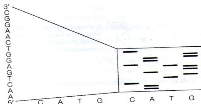
Fig. 3. Motif en échelle obtenu après séquençage d'ADN et électrophorèse.
