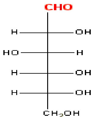
ALDOSE
