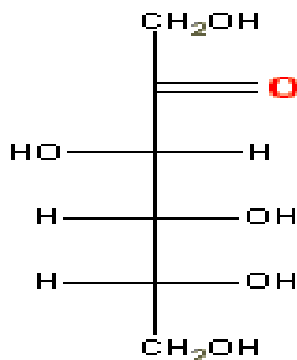
CETOSE
