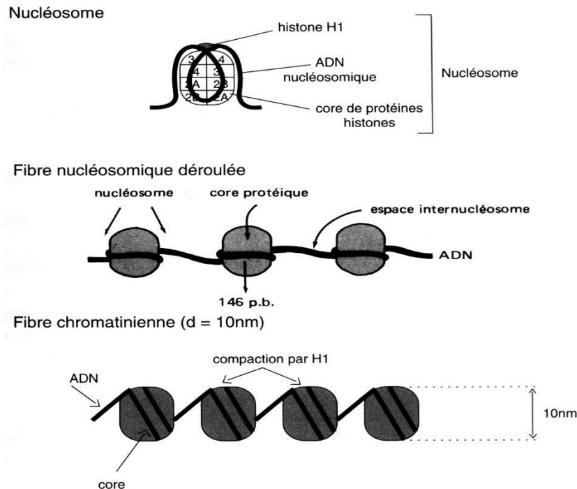
Figure 9.2 : Unité chromatinienne.
