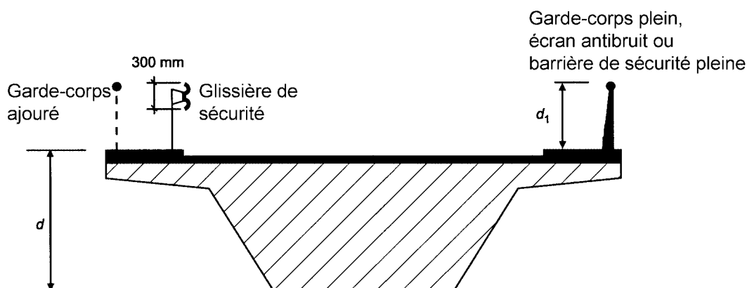
Figure 8.5 — Hauteur à prendre en compte pour A_{ref,x}
