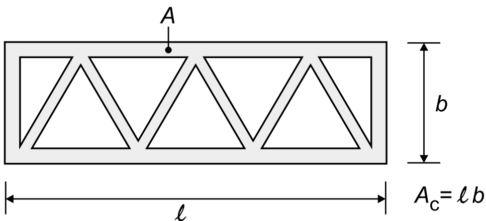
Figure 7.37 — Définition du taux de remplissage \varphi
