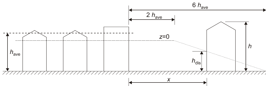
Figure A.5 — Hauteur d'obstruction et espacement au vent
