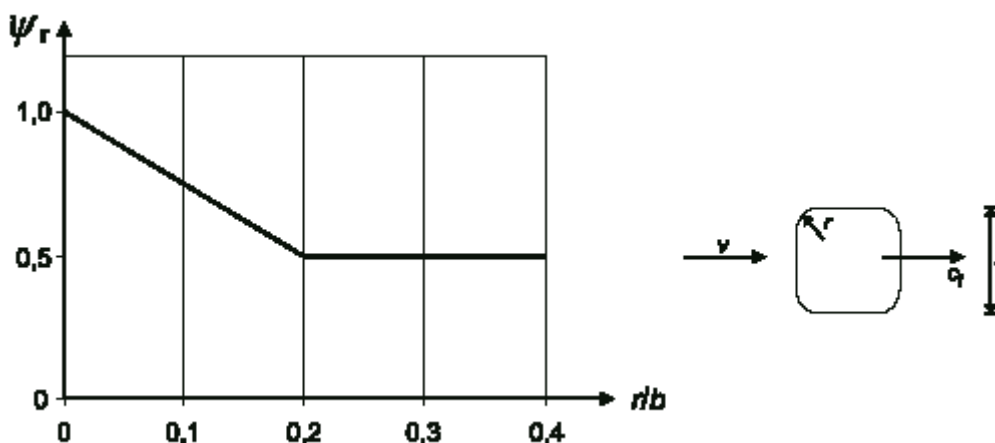
Figure 7.24 — Facteur de réduction \psi_r pour une section transversale carrée à angles arrondis
