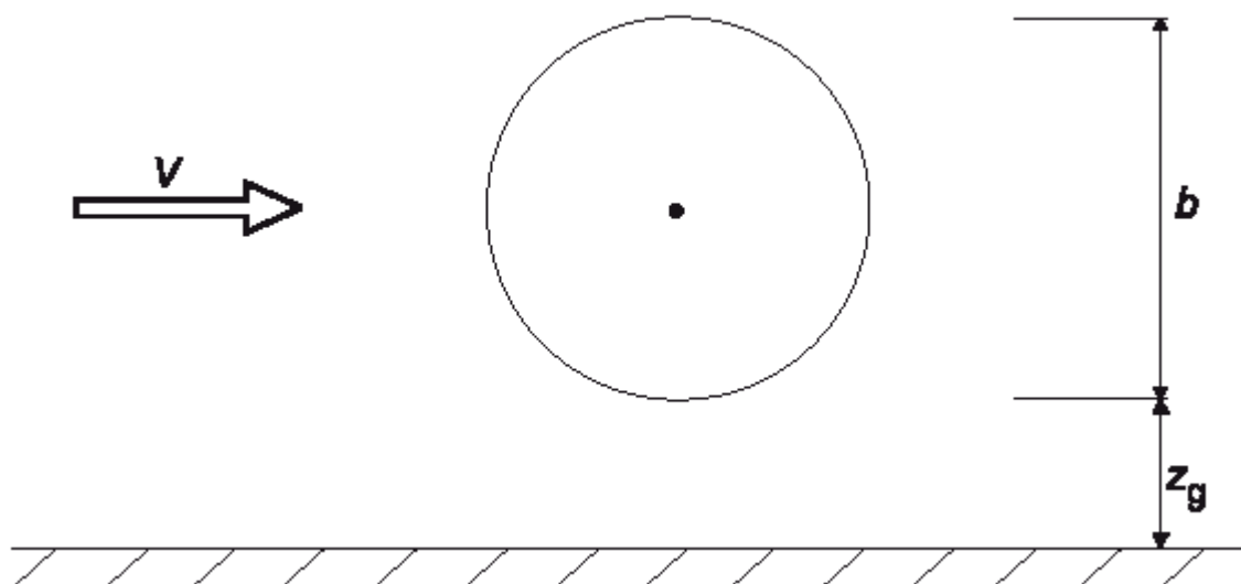
Figure 7.29 — Cylindre proche d'une surface plane
