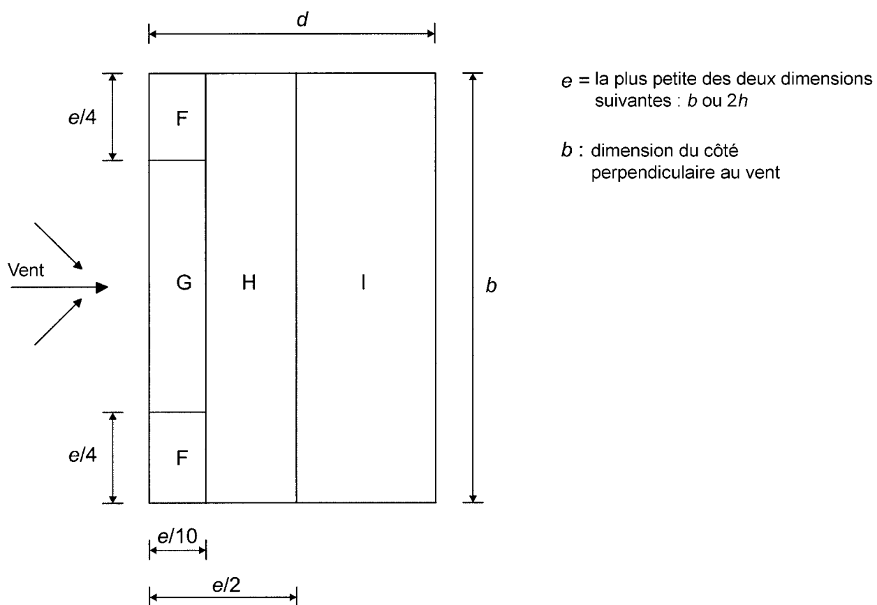
Figure 7.6 — Légende applicable aux toitures-terrasses
