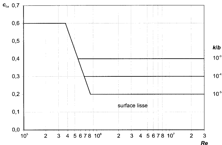
Figure 7.30 — Coefficient de force d'une sphère dans le sens du vent
