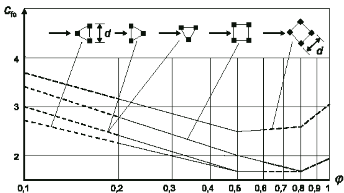
Figure 7.34 — Coefficient de force c_{f,0} d'une structure spatiale en treillis composée de profilés en fonction du taux de remplissage \phi
