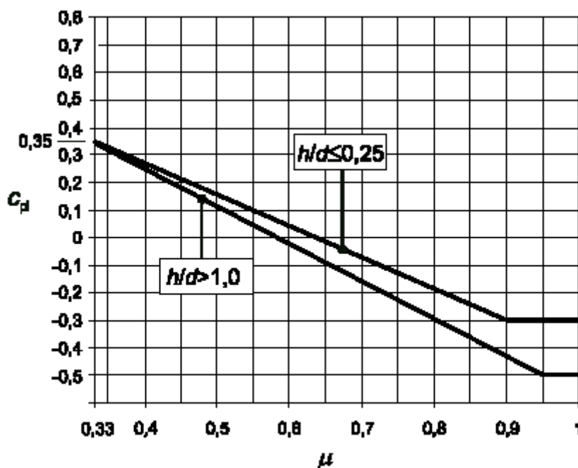
Figure 7.13 — Coefficients de pression intérieure applicables pour des ouvertures uniformément réparties
