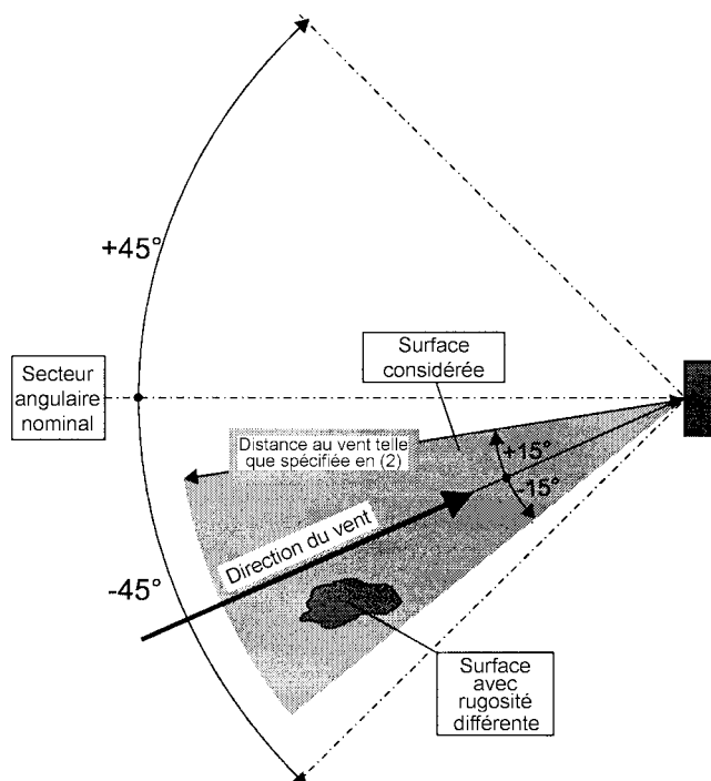
Figure 4.1 — Évaluation de la rugosité du terrain
