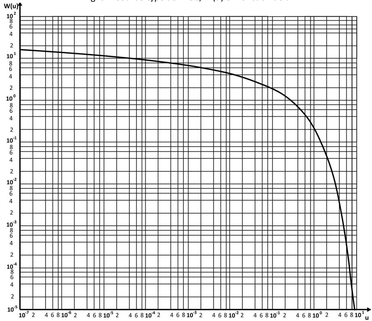
Fig. 02- Courbe-type de Theis, W(u) en fonction de u
